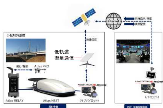
図-2 AtlasNEST の機材構成図（小松川斜張橋）
