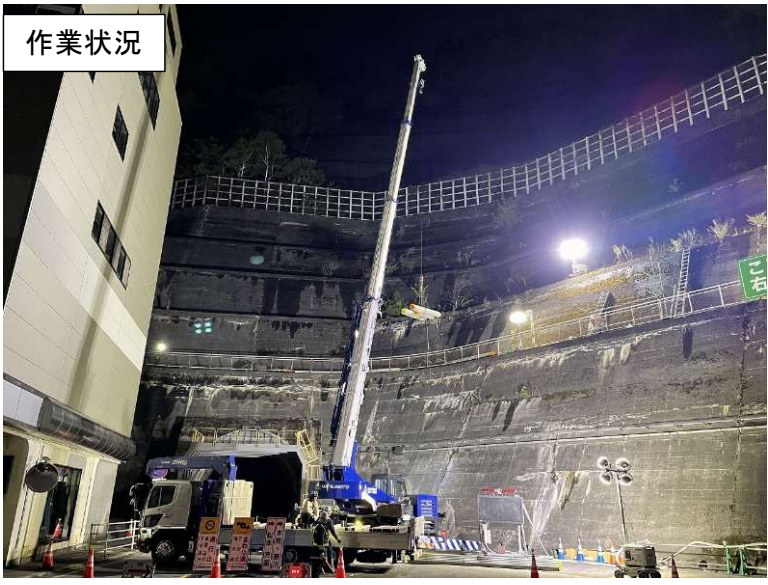
新入山隧道坑口部 法面補強工
