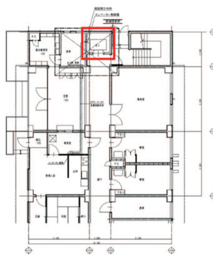
(新設)1階平面図
