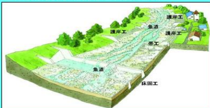
護岸工
