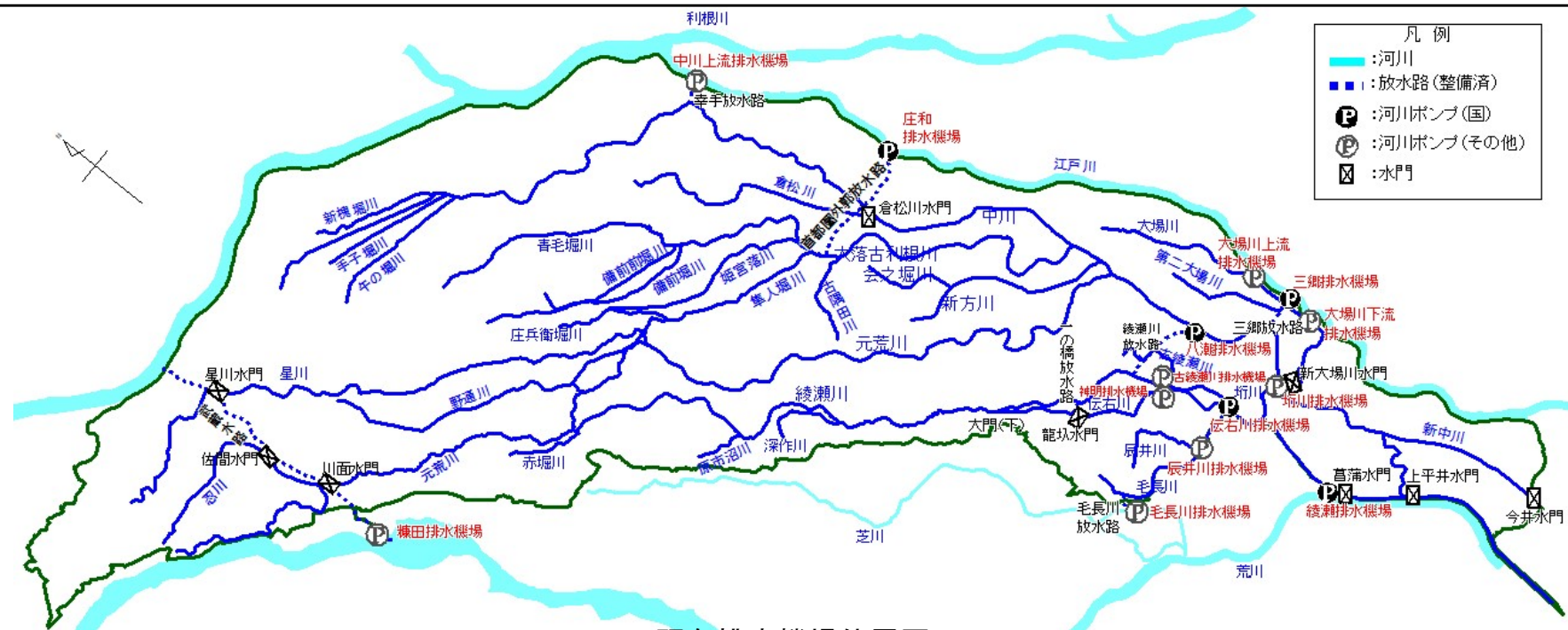
既存排水機場位置図
