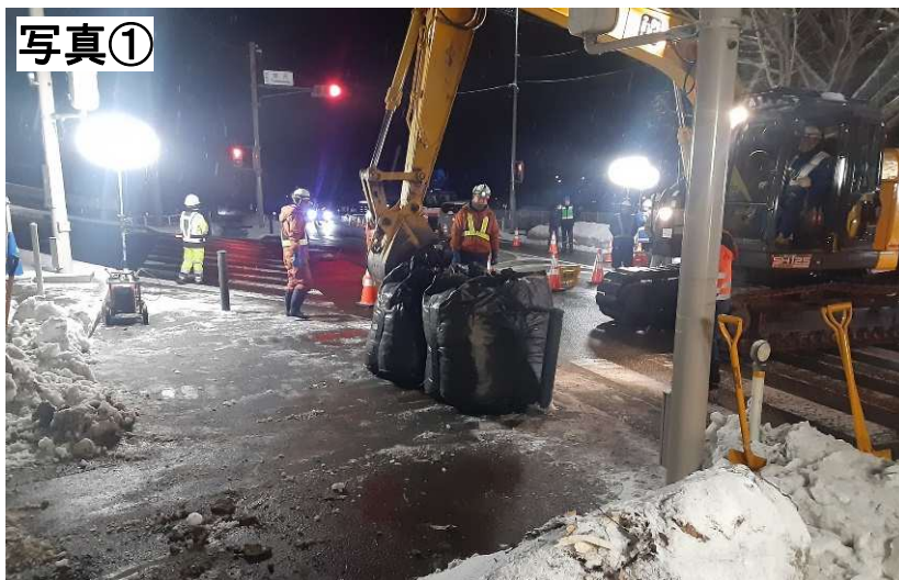
大型土のう設置状況①
