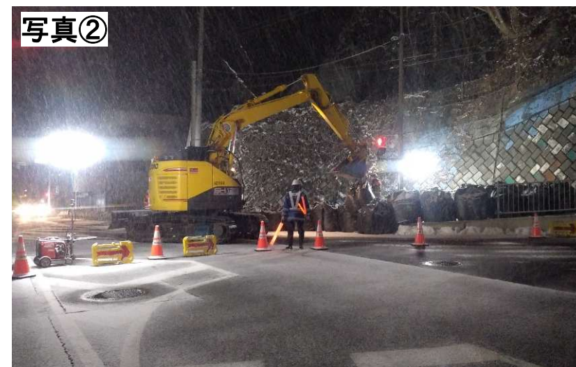
大型土のう設置状況②
