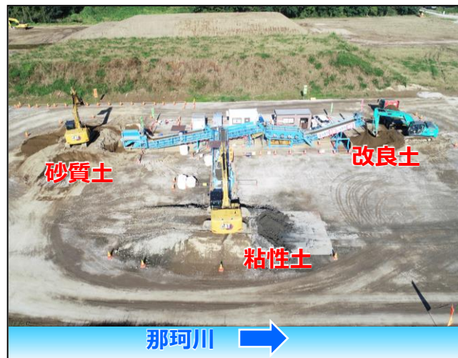
土砂改良プラント (城里町下阿野沢地先)
