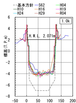
鶴見川河床横断重図
