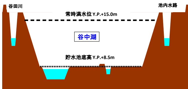
干し上げ期間(水位 Y.P.+8.5m -20cm)の 貯水池断面イメージ
