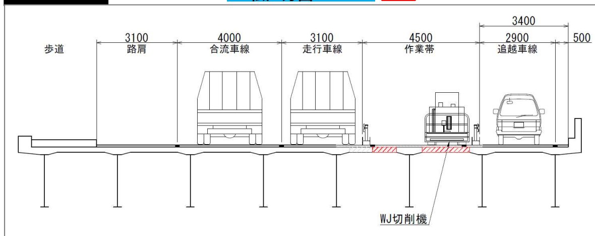
A-A断面図
