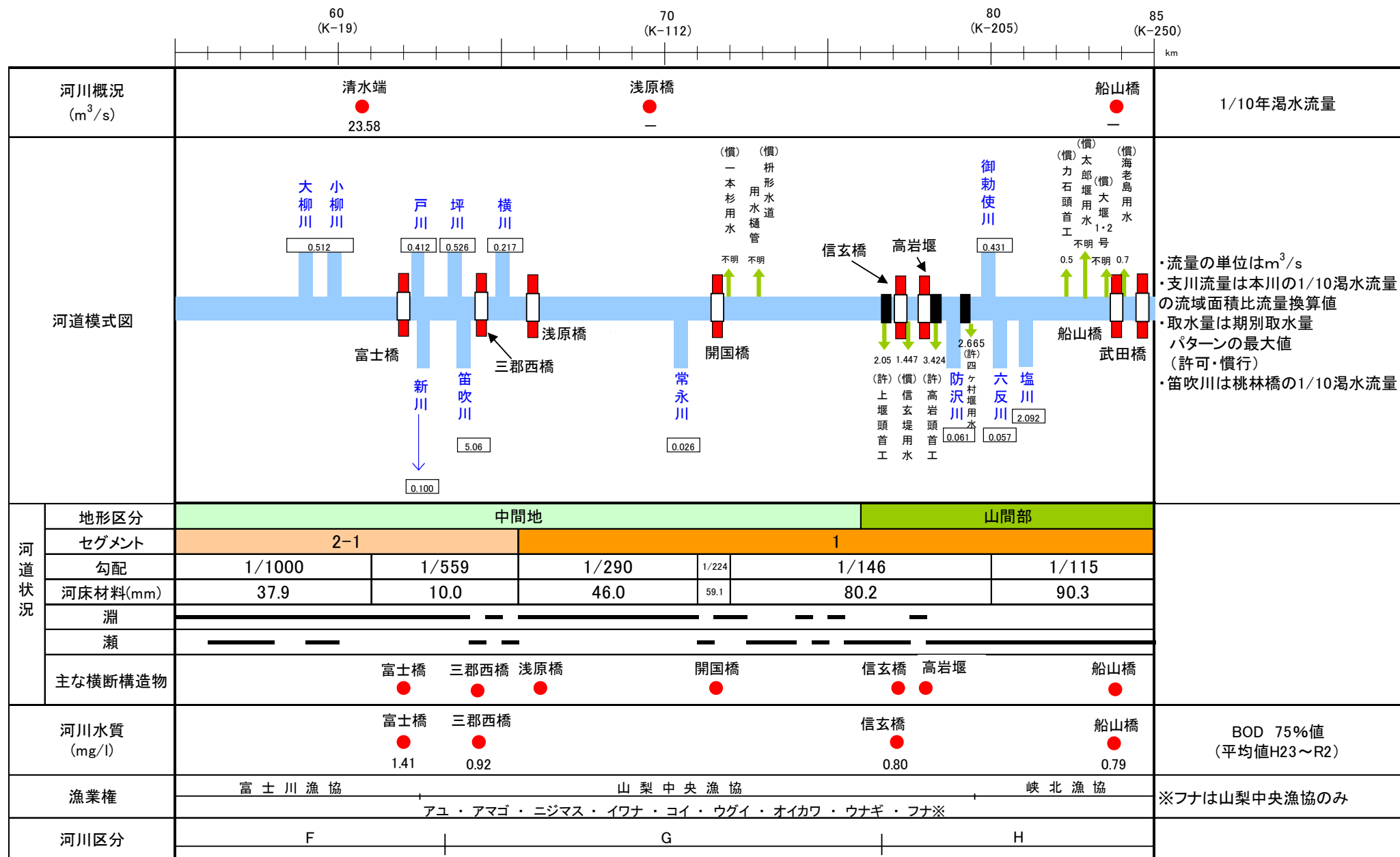
図2-3 河川環境の縦断特性(釜無川)
