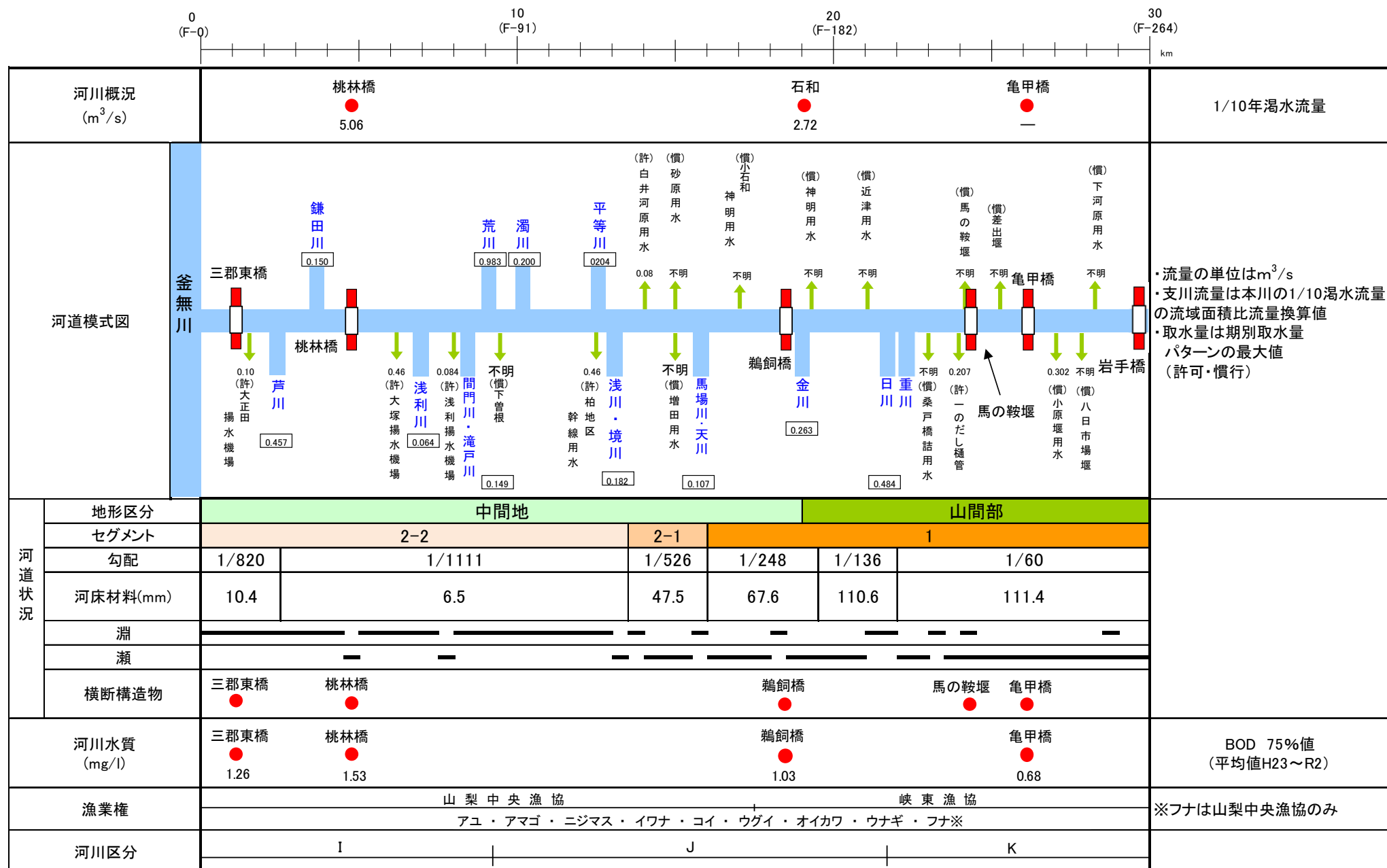
図2-4 河川環境の縦断特性(笛吹川)
