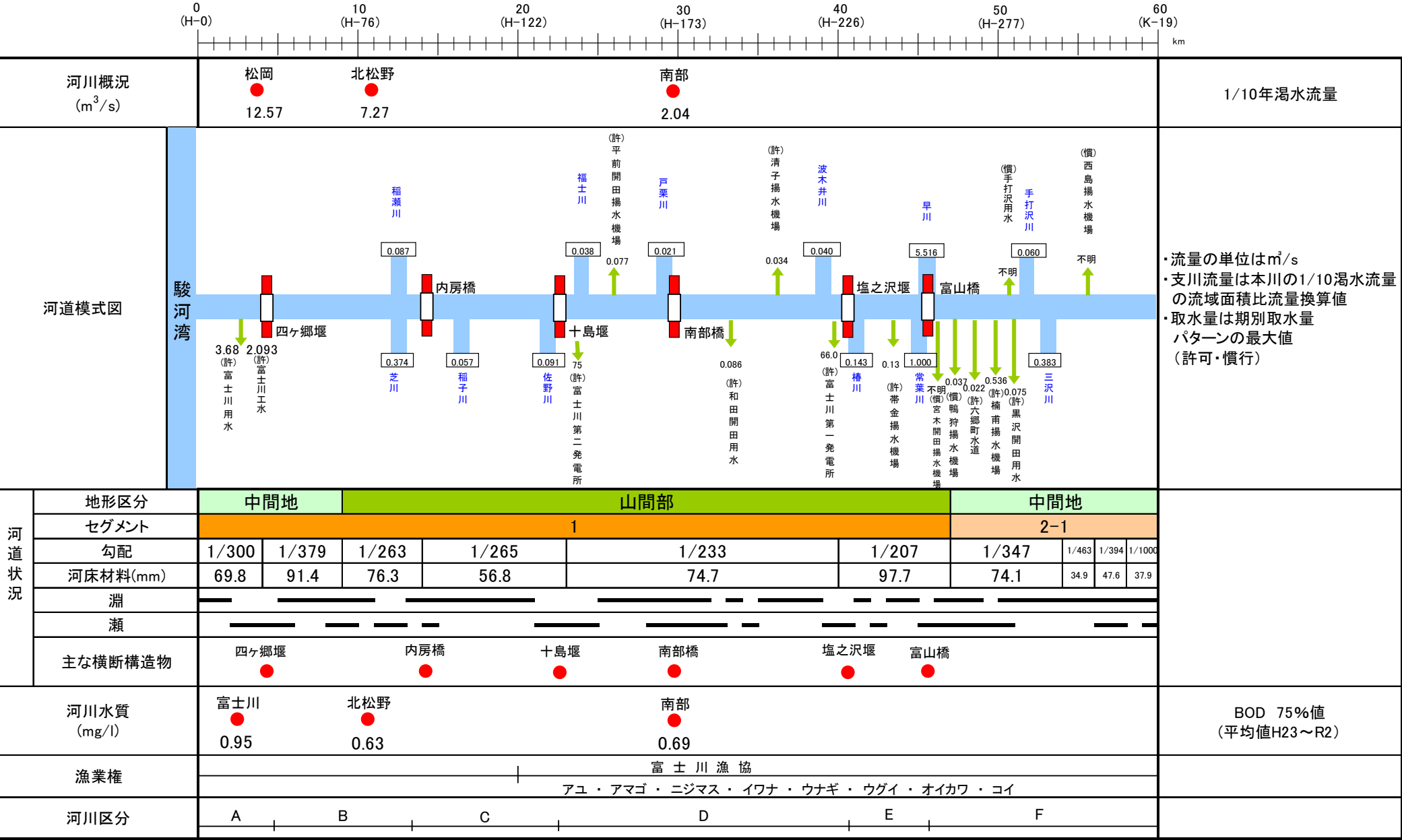
図2-2 河川環境の縦断特性(富士川)
