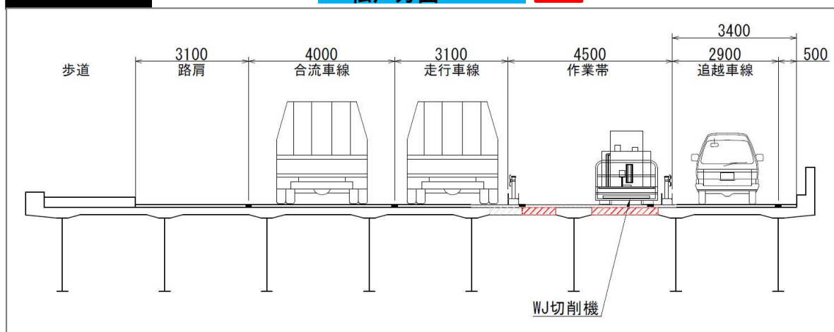
A - A 断面図
