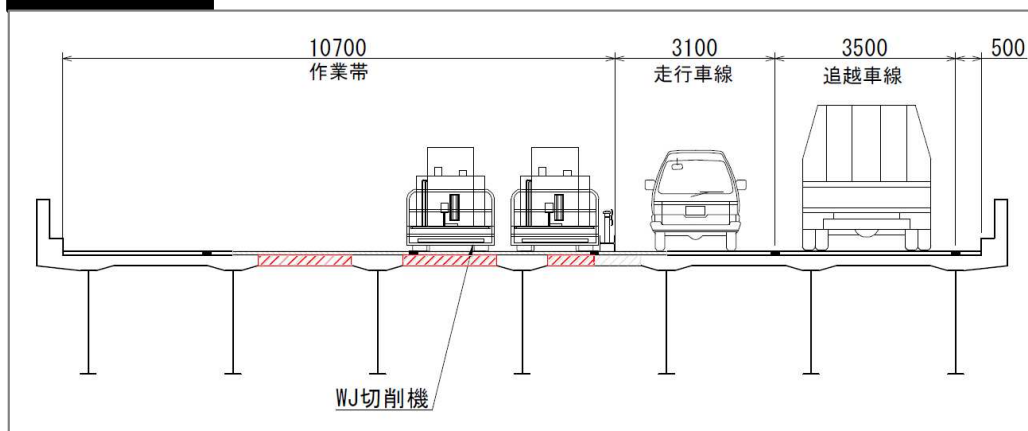
A-A断面図
