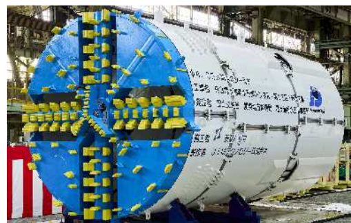
掘削前のシールドマシン
