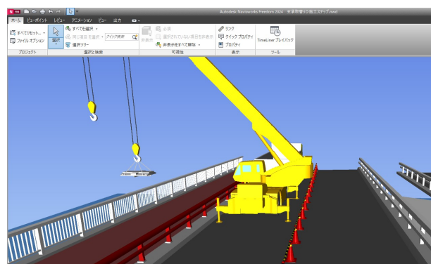
図-1 3次元施工ステップ（車線規制）
