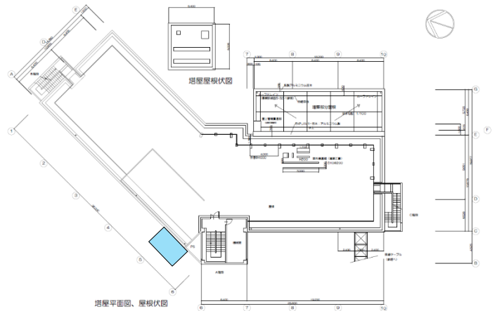
屋上平面図
