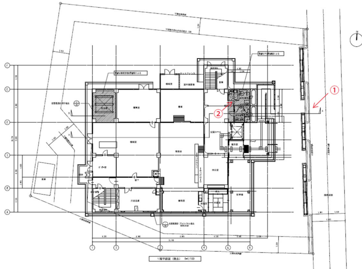
配置図・1階平面図
