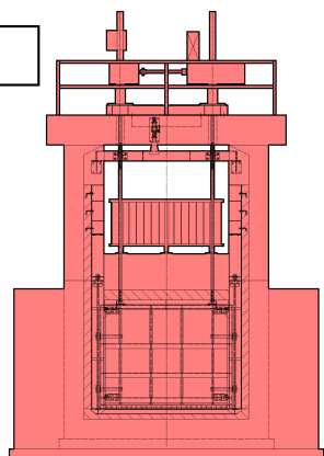
桶管正面図
