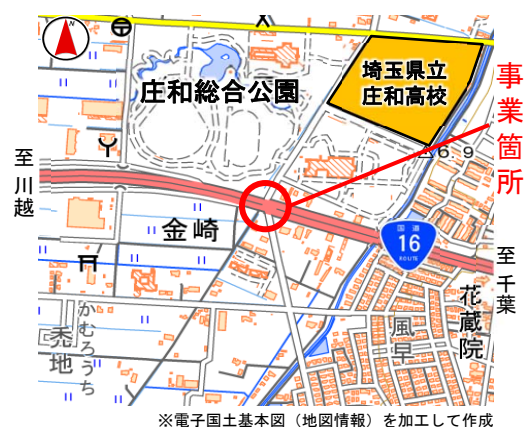
【詳細図】
