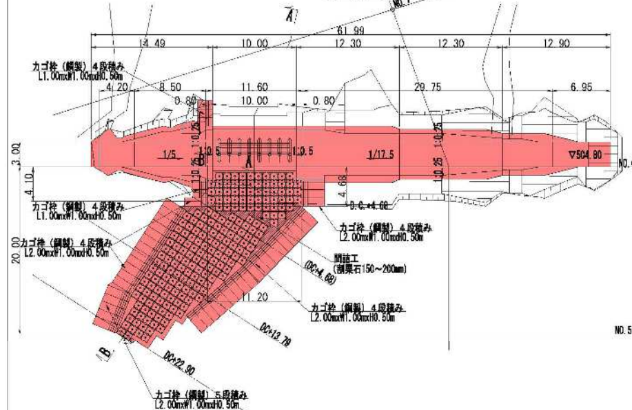
平面図
