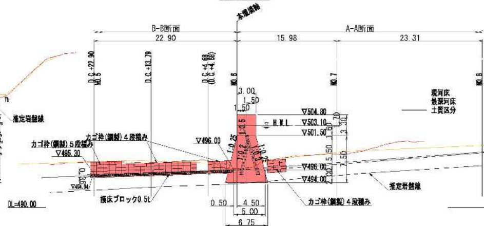
側面図
