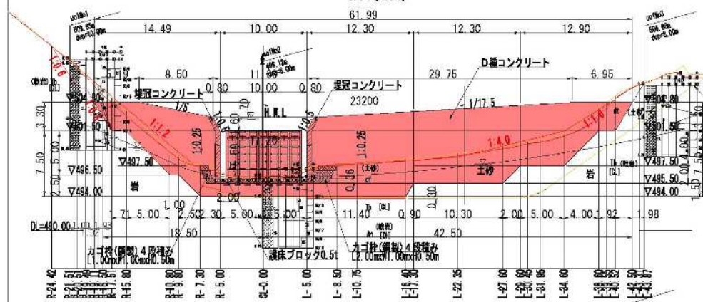
本堤工正面図 P.1 (NO.6)
