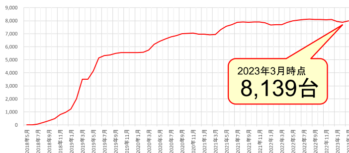
危機管理型水位計台数推移(2023年3月末時点)
