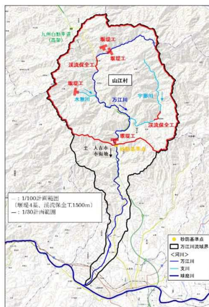
土砂・洪水氾濫対策の施設配置図
