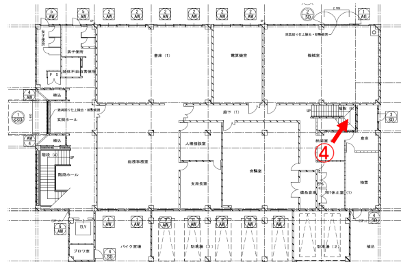
1階平面図
