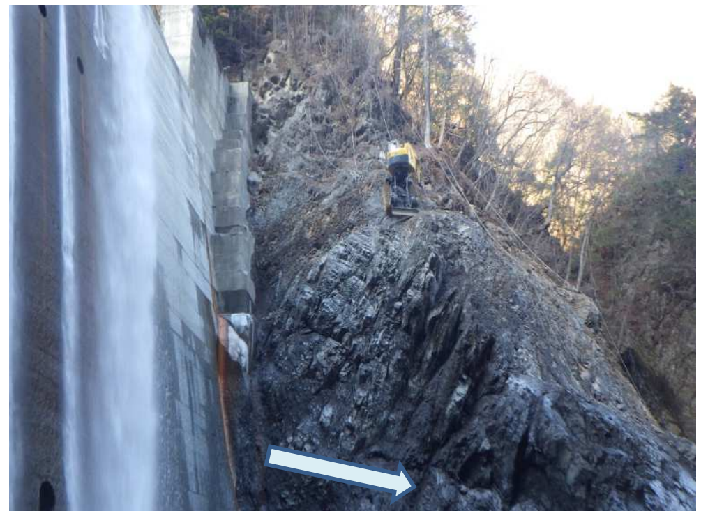
対岸より施工箇所を望む
