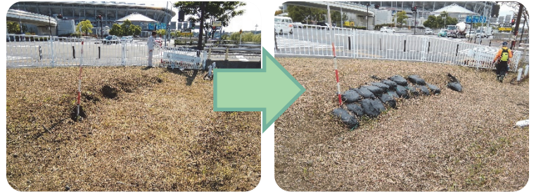
堤防の法面の補修前後
