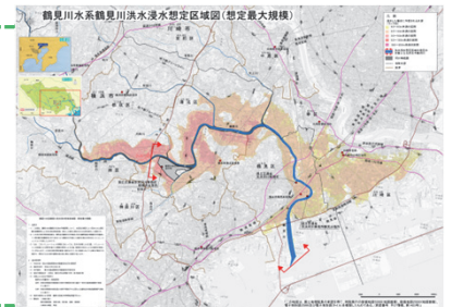
鶴見川洪水浸水想定区域図
