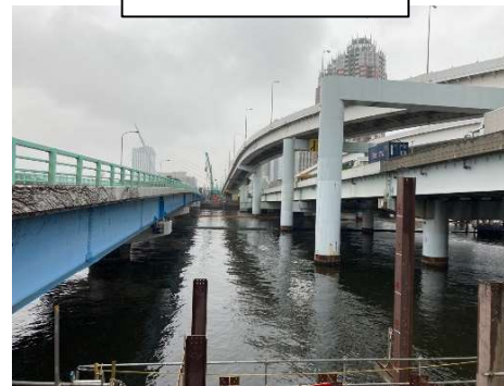
③UP16,UP15橋脚
