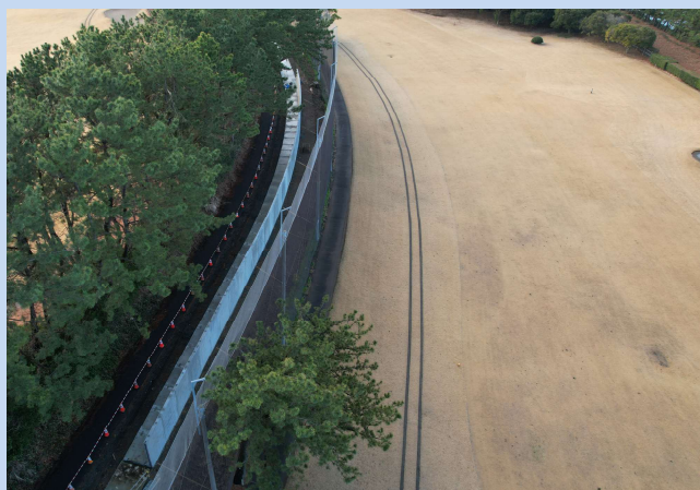
擁壁を設置しています。 (令和6年2月)
