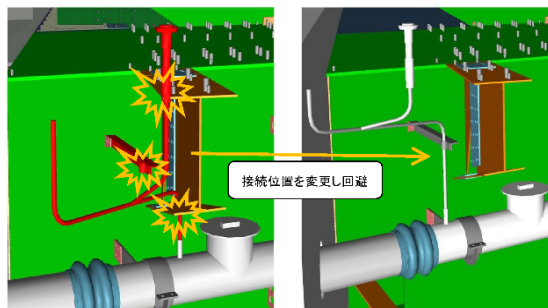
S1 ブラケットとスラブドレーン管の干渉確認
