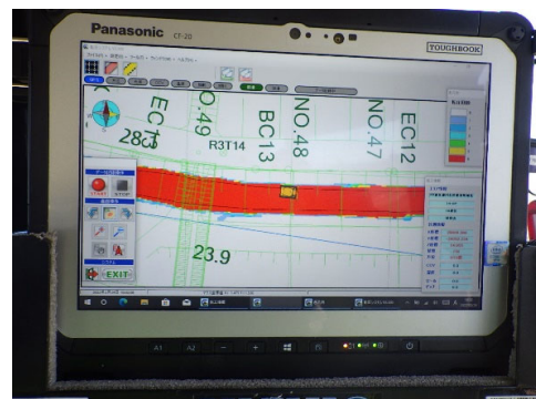
盛土締め ICT建機の確認モニター
