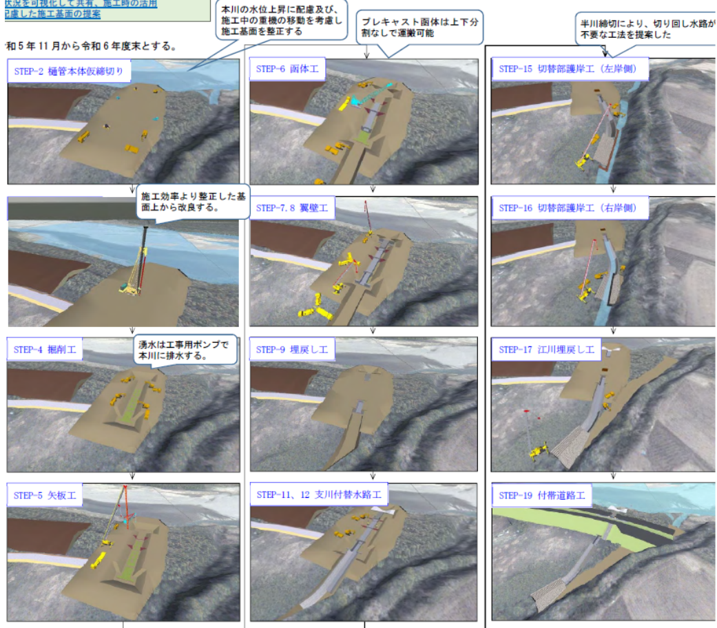
図2 施工ステップモデル (抜粋)
