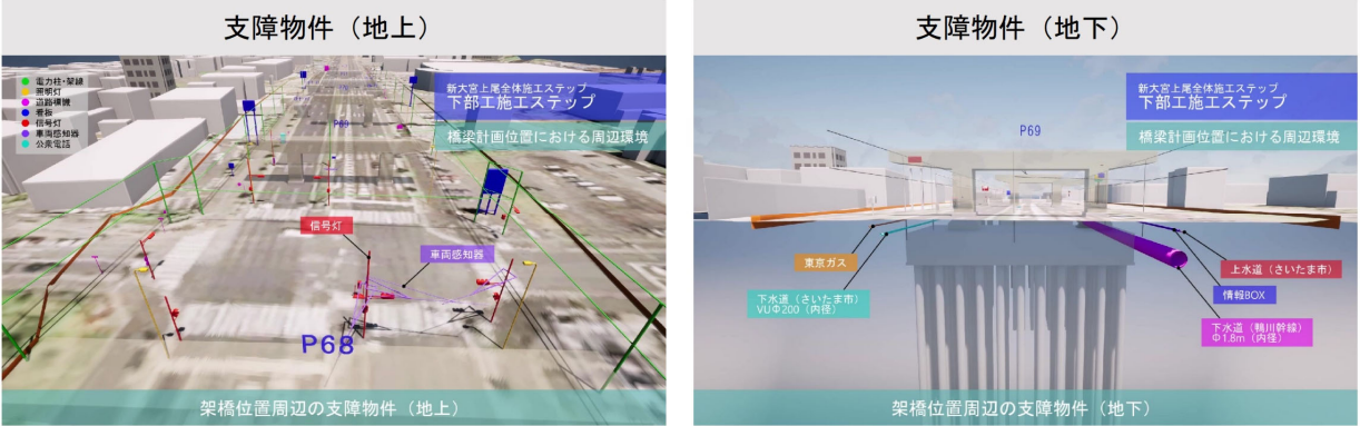
図1 支障物件（地上及び地下）の視覚的な
