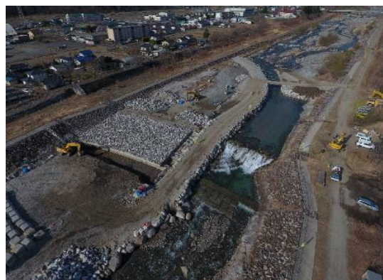
右岸側石組 施工状況
