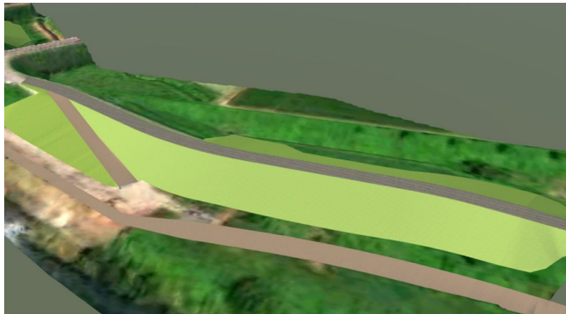
施工ステップ（築堤後）
