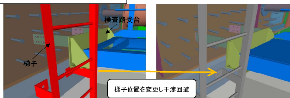
S1 橋桁付き検査路受台と梯子の干渉確認
