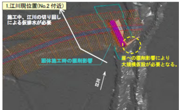
図-1 配置検討に使用した CIM モデル(江川現位置)
