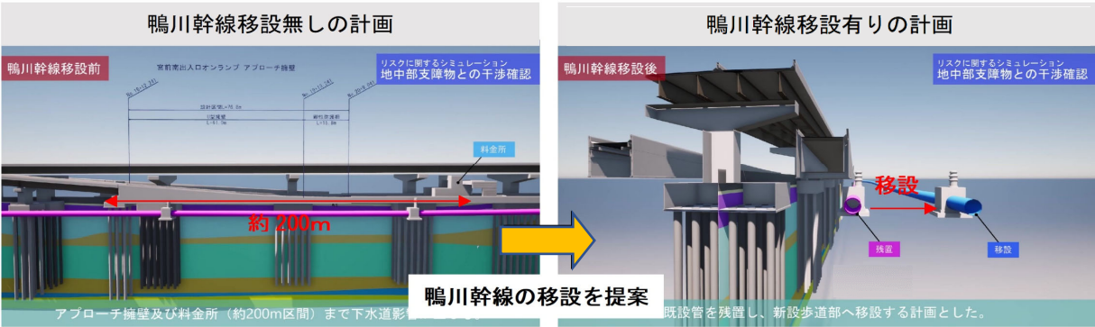
図3 橋梁と幹線下水道との近接・干渉状況の可
