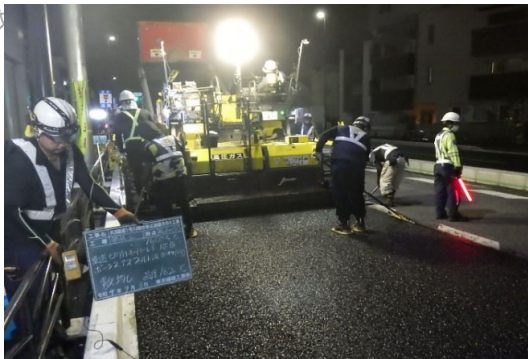
車道舗装 施工状況
