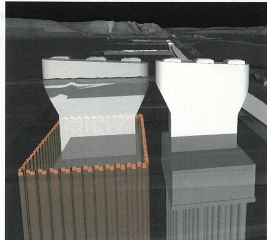
II期施工時におけるI期施工下部構造との 近接施工の妥当性確認
