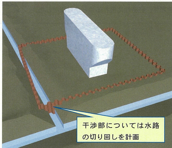
地下埋設物との取り合い確認
