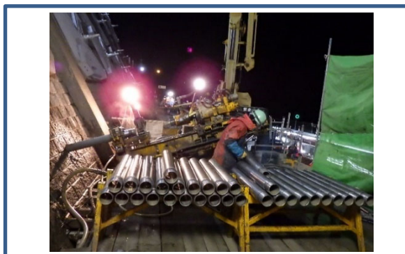
アンカー施工状況
