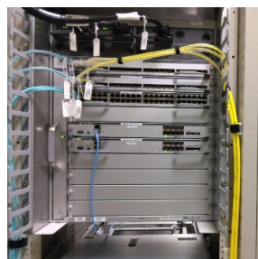
伝送機器設置状況
