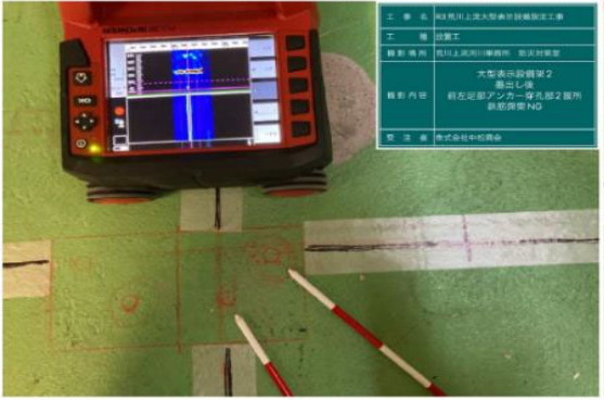
鉄筋探索NG状況
