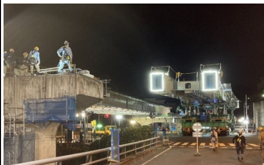
多軸台車一括架設状況
