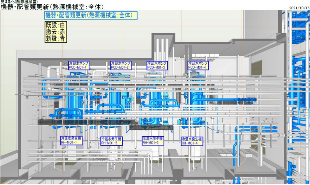
機械室見下げ図 新設後
