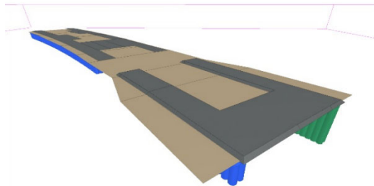
3次元設計データ 基盤整備工(土工)
