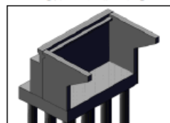
【背面（A2橋台）】
