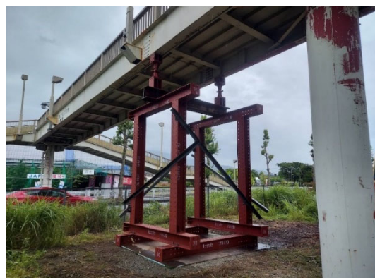
仮バント設置完了状況
