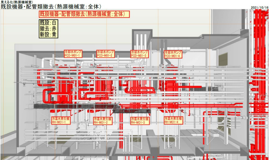
機械室見下げ図 撤去前
