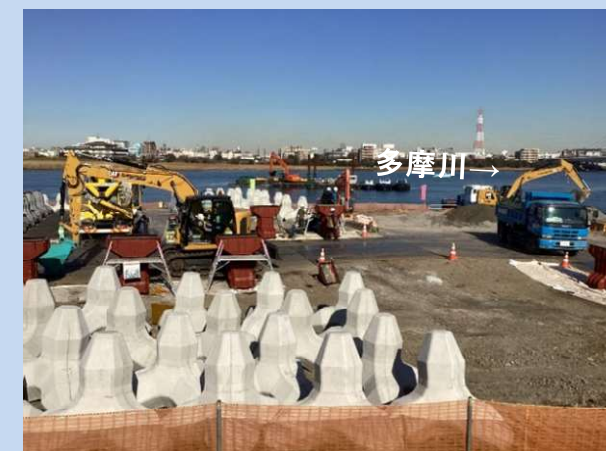
根固めブロックを製作しています。 (令和5年12月)
