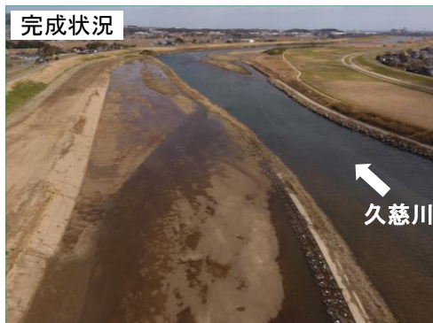
R3久慈川左岸下土木内町地先下流河道掘削外工事 (増子建設株式会社)
