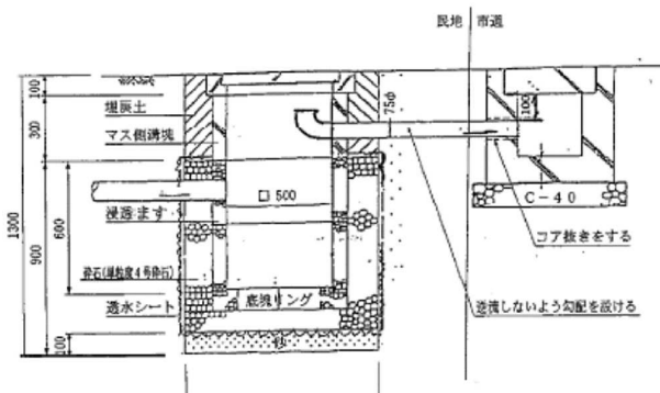
浸透枳構造図
