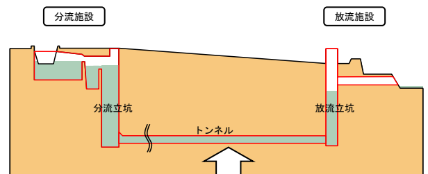
五反田川放水路を雨水貯留施設として活用
