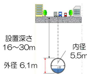
分水路断面图
