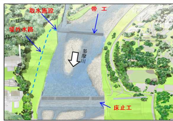
大丸用水堰改築のイメージ
