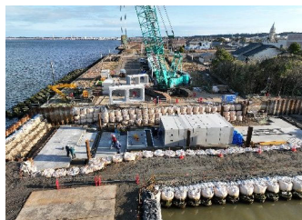
【巨大なメガネ据付中！】 岡田土建(株) 小倉 隼人
