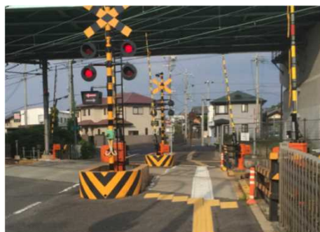
(踏切手前への視覚障害者誘導用ブロック、踏切内への誘導表示を設置した事例)
