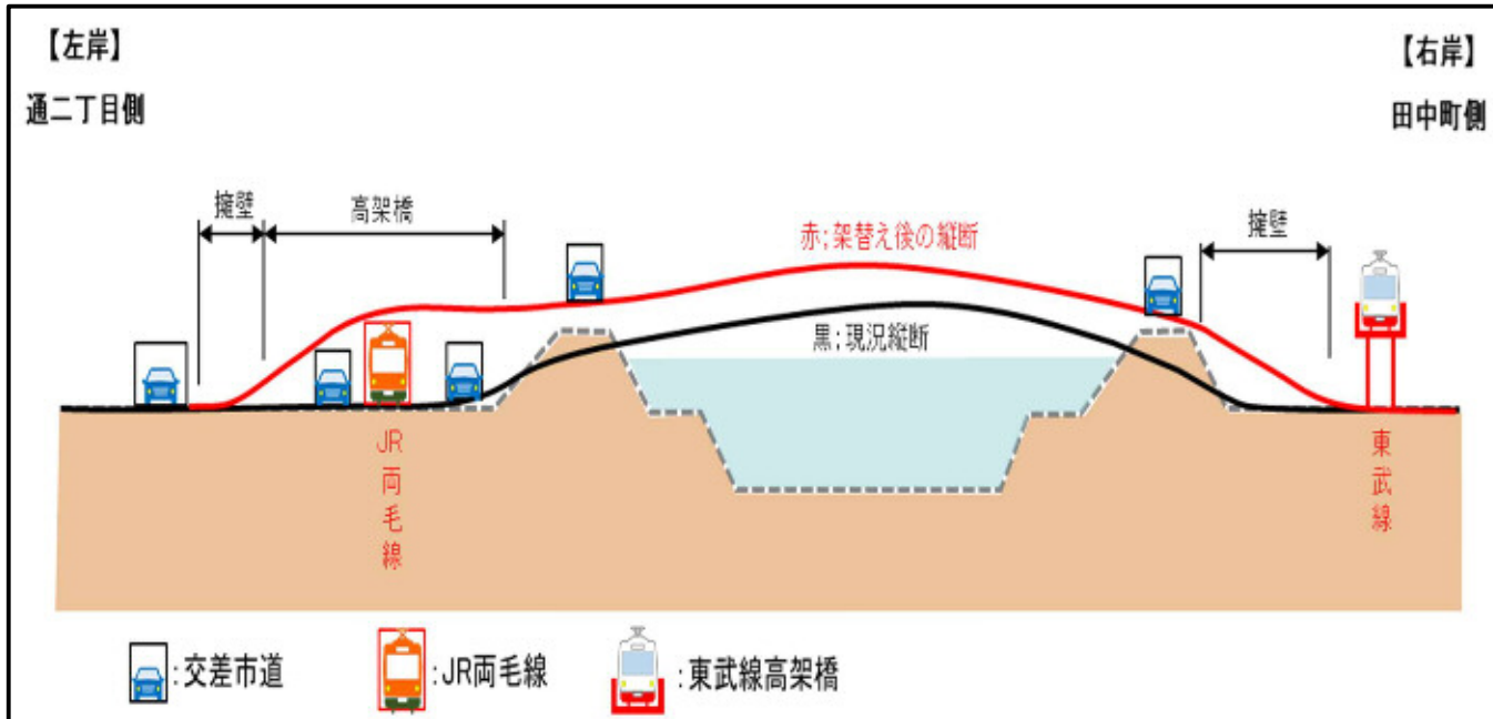
【中橋架替縦断線形イメージ】
