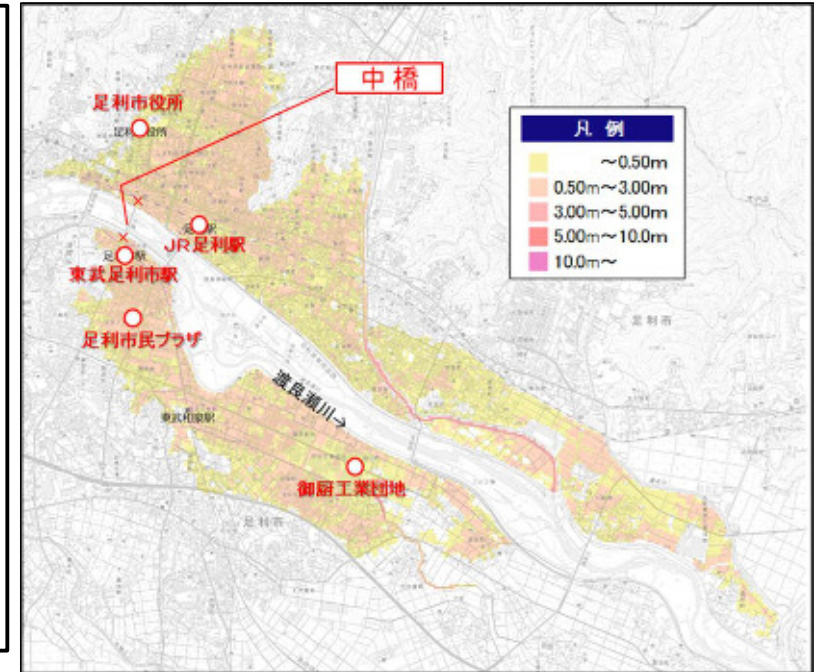
【計画規模洪水による氾濫シミュレーション浸水図】
