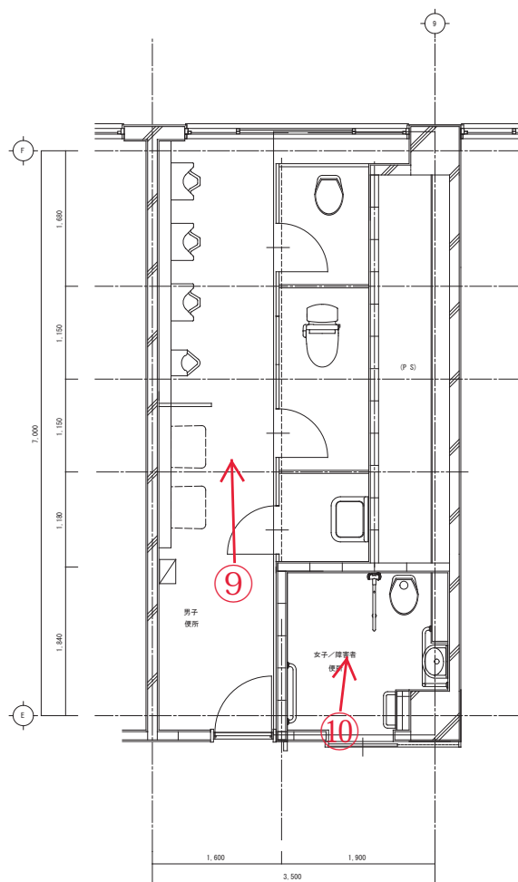
1階 便所詳細図
