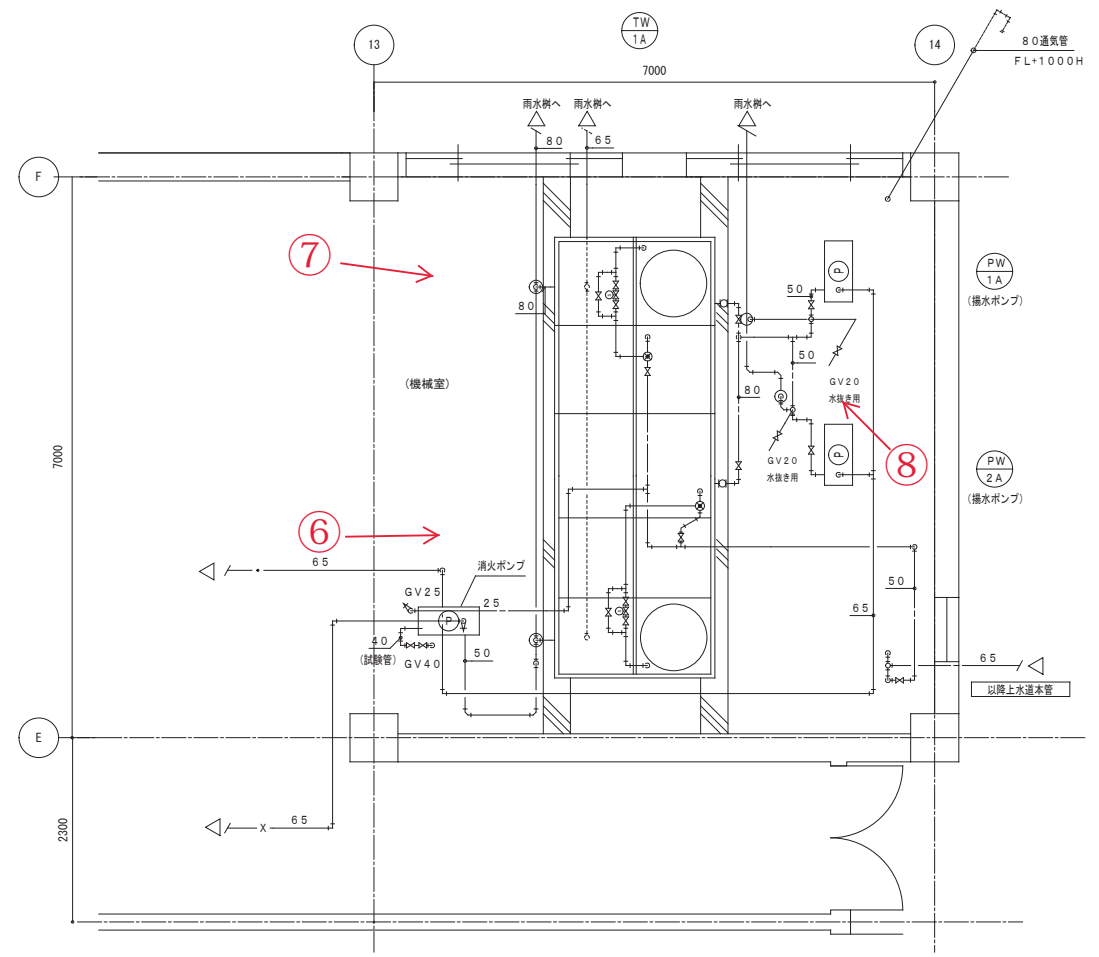
受水槽廻り
