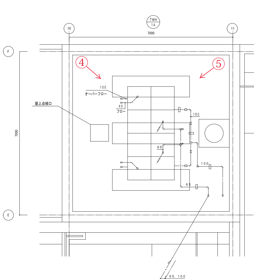
高置水槽廻り
