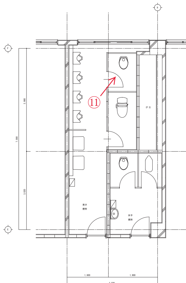
2階 便所詳細図
