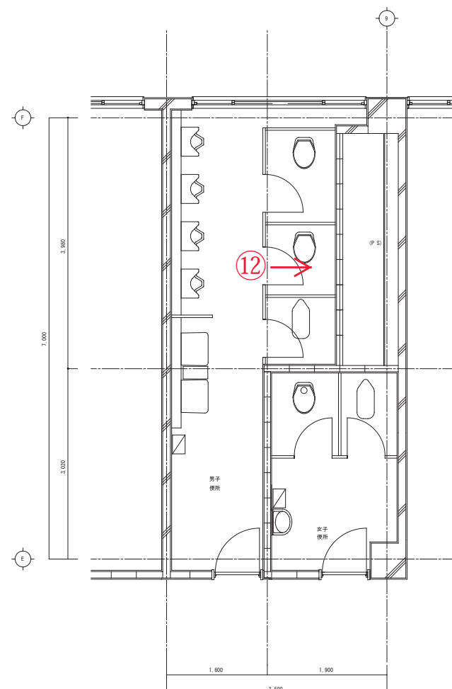
3階 便所詳細図
