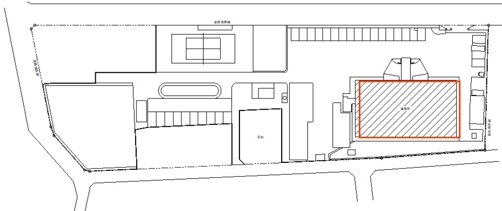
配置図
