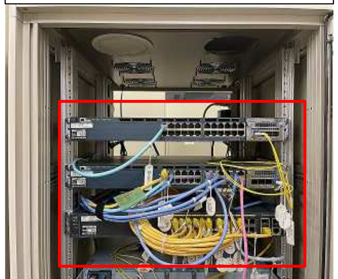
ネットワーク設備設置状況 (北千葉第二機場)
