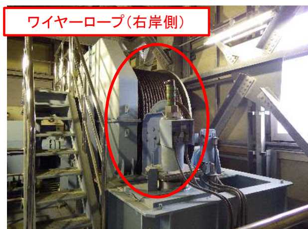
ワイヤーロープ(交換対象)
