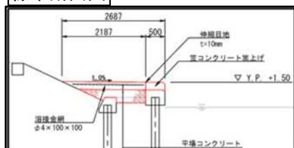
標準断面図
