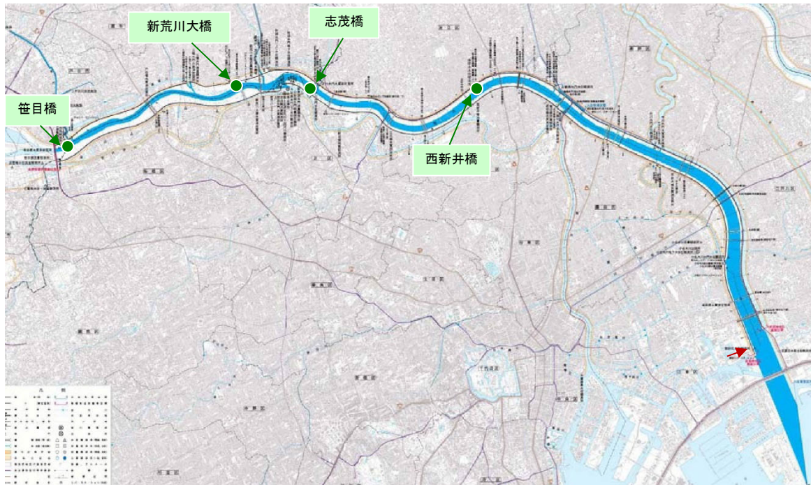
図-5 高水流量観測所位置図
