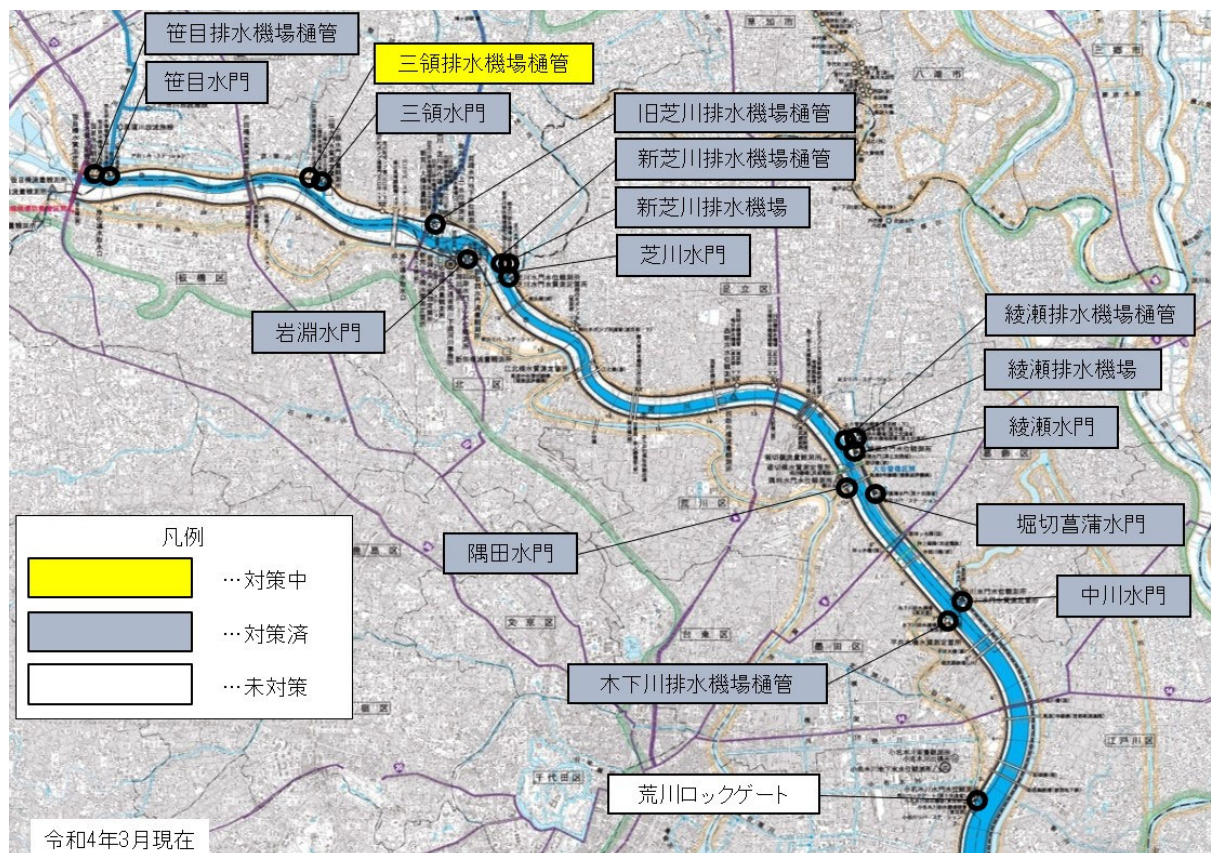
図 3-2 レベル2地震動に対する耐震対策の必要な施設と対策状況
