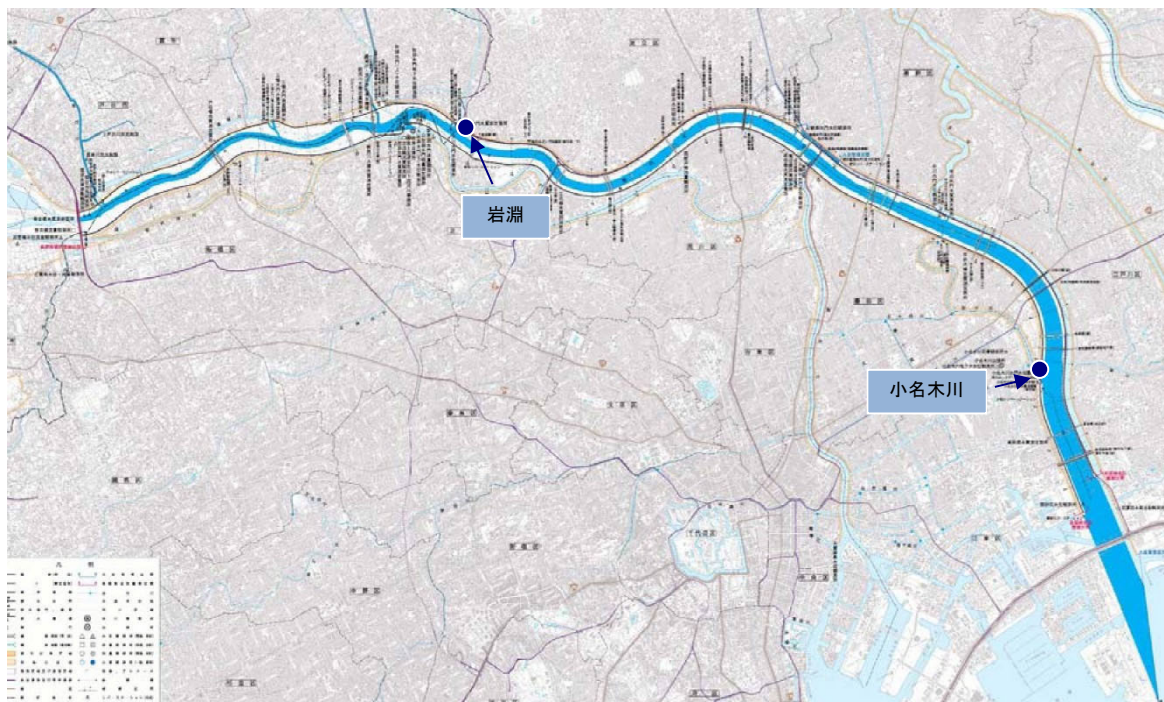
図一1 雨量観測所位置図(荒川)
