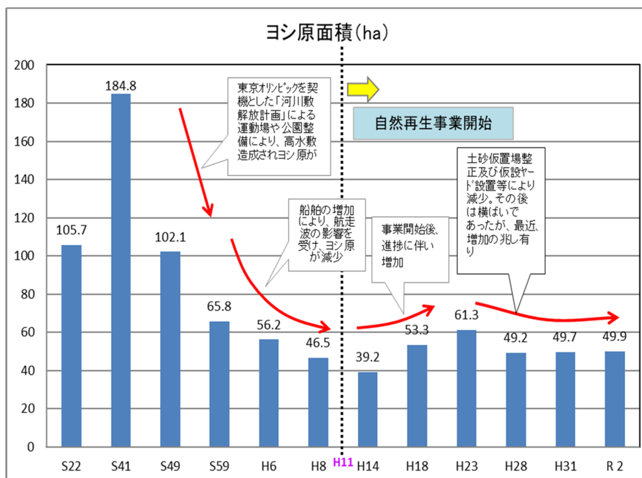
図 3-6 河岸の侵食とヨシ原の変化
