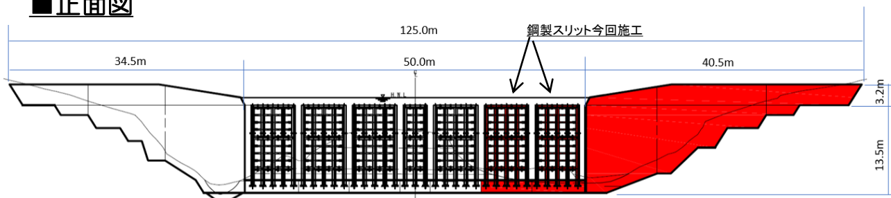
■正面図
