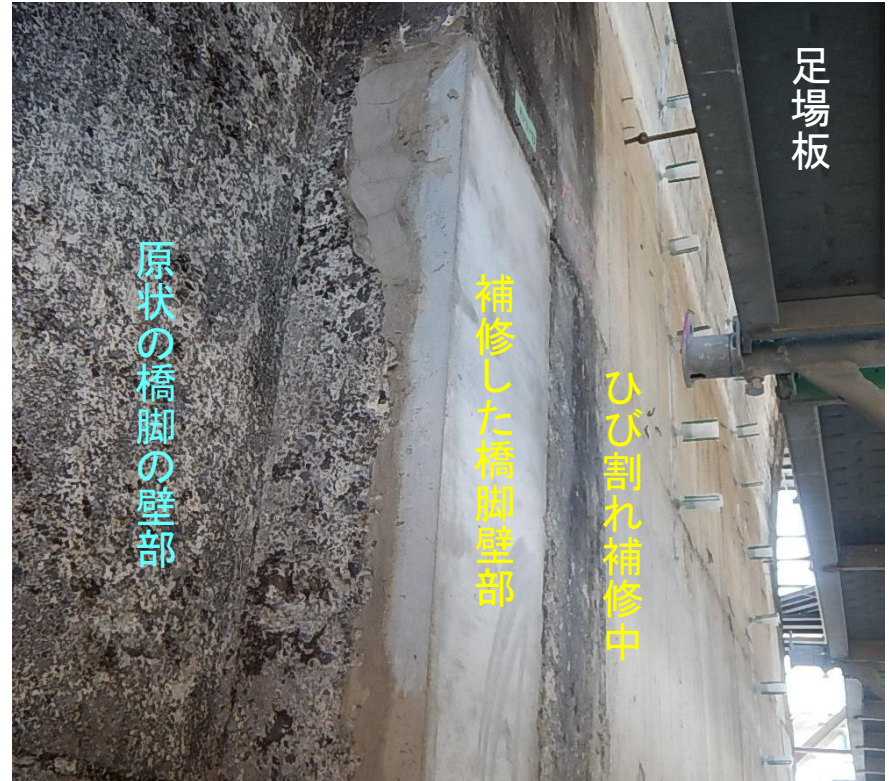
橋脚柱(壁)部の補修状況
