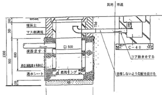
浸透樹構造図
