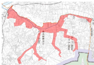
江川流域環境保全対象箇所
