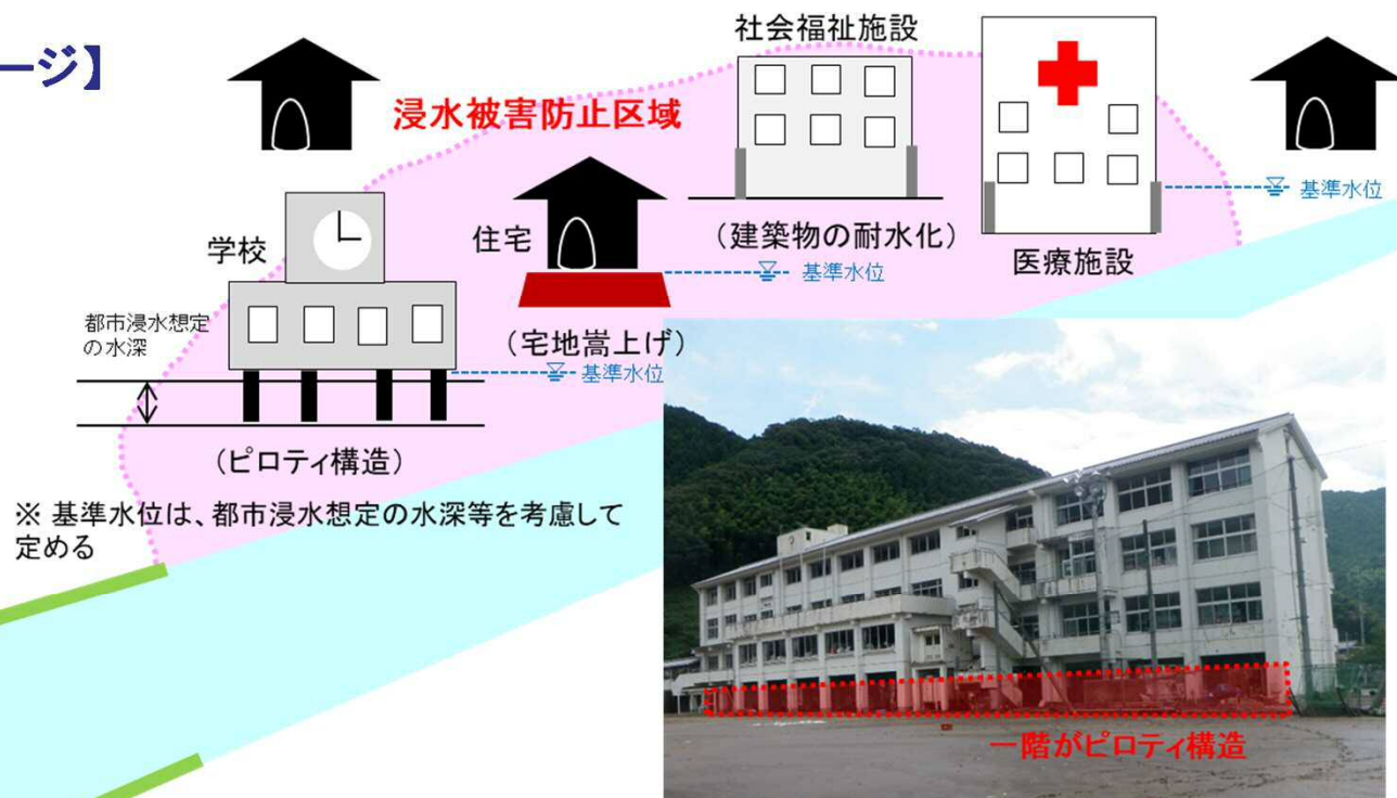
ピロティ構造の事例
