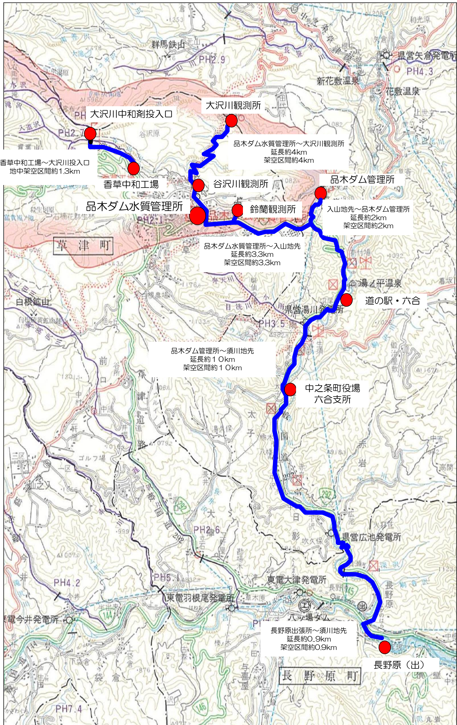
別図-1 品木ダム電気通信設備図
