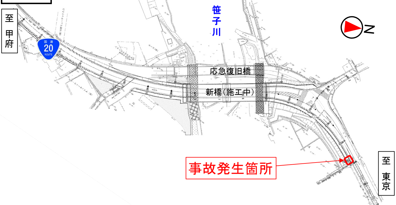
詳細位置
