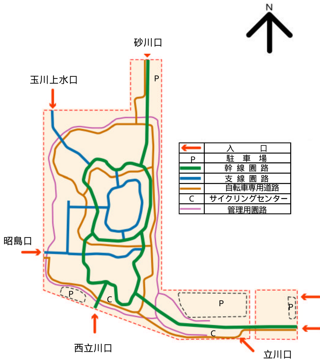
動線計画図
