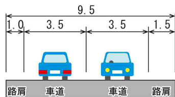
横断面図
