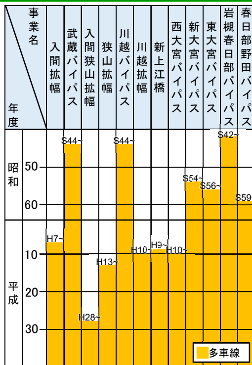
埼玉県内の国道16号の多車線化事業
