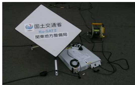
Ku-SAT II (可搬式衛星通信装置)
