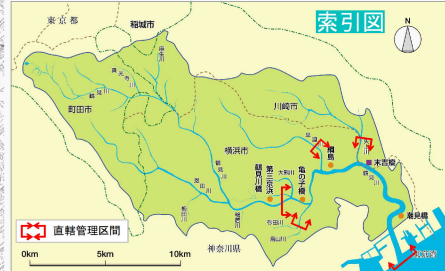
鶴見川水系洪水浸水想定区域図(計画規模)
