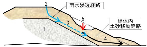
図-3 “陥没”の発生要因想定（例）
