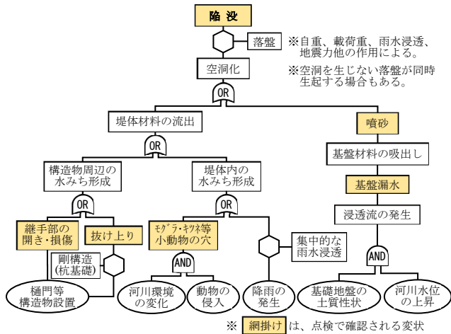
図-2 堤防の変状（陥没）に関するFT図（例）
